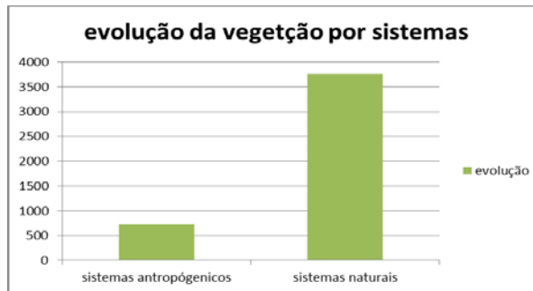
Gráfico 4. Evolução da vegetação por sistemas
